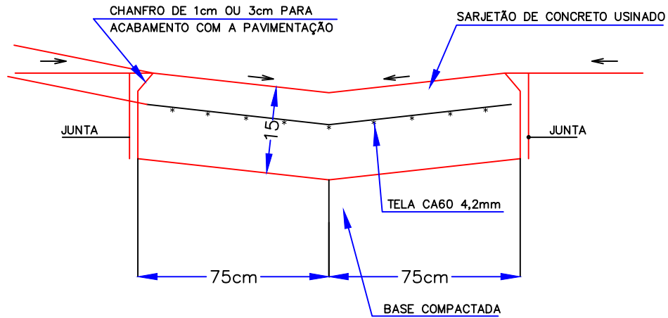
CORTE SARJETÕES PAVIMENTAÇÃO S/ESC.
