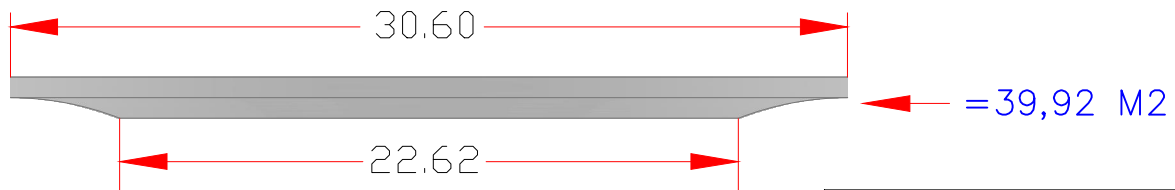
DIMENSÕES SARJETÕES PAVIMENTAÇÃO S/ESC.
