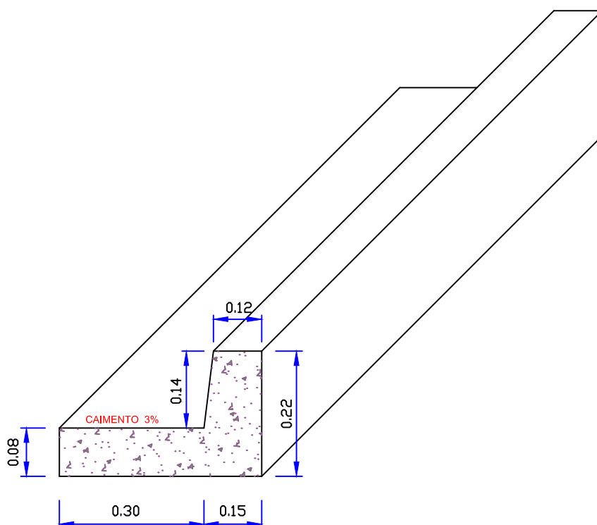
DETALHE GUIAS E SARJETAS S/ESC.
