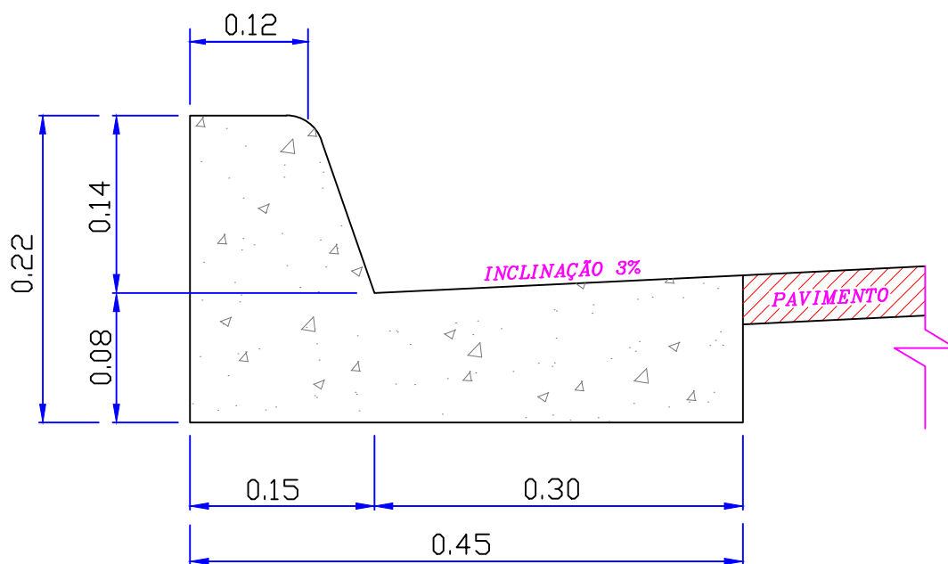
CORTE GUIA A SARJETA S/ESC.
